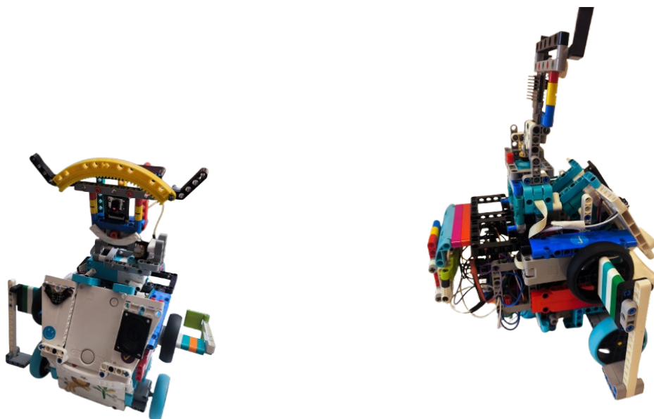
Figura 4.1: Robotul TriSense în configurația finală: vedere frontal-oblică (stânga) și laterală (dreapta).
