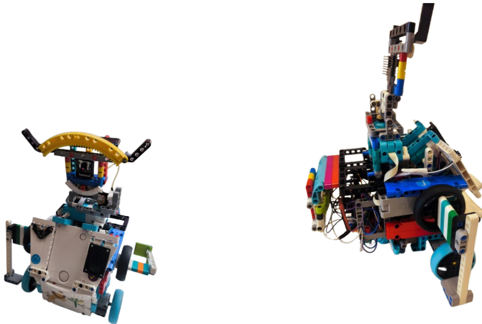
Figura D.1: Robotul TriSense în configurația fizică finală: vedere frontal-oblică (stânga) și laterală (dreapta).
