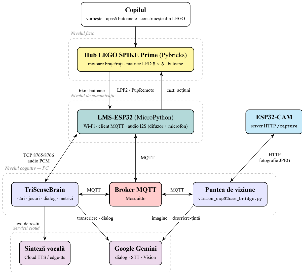
Figura C.1: Arhitectura logică a sistemului TriSense: cele trei niveluri de execuție (hub LEGO, LMS-ESP32, PC), modulul ESP32-CAM și serviciile cloud, împreună cu protocoalele de comunicație dintre ele.
